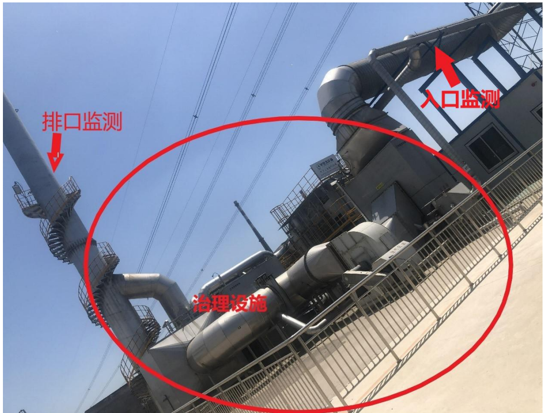
图 4-1 比较规范的采样位置设置图
